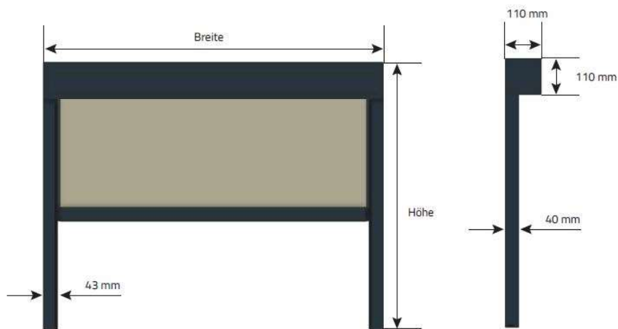
Abbildung 1: Breite und Höhe der Senkrechtmarkise
